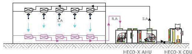
수직 층류방식(class 100 ~ 0)
